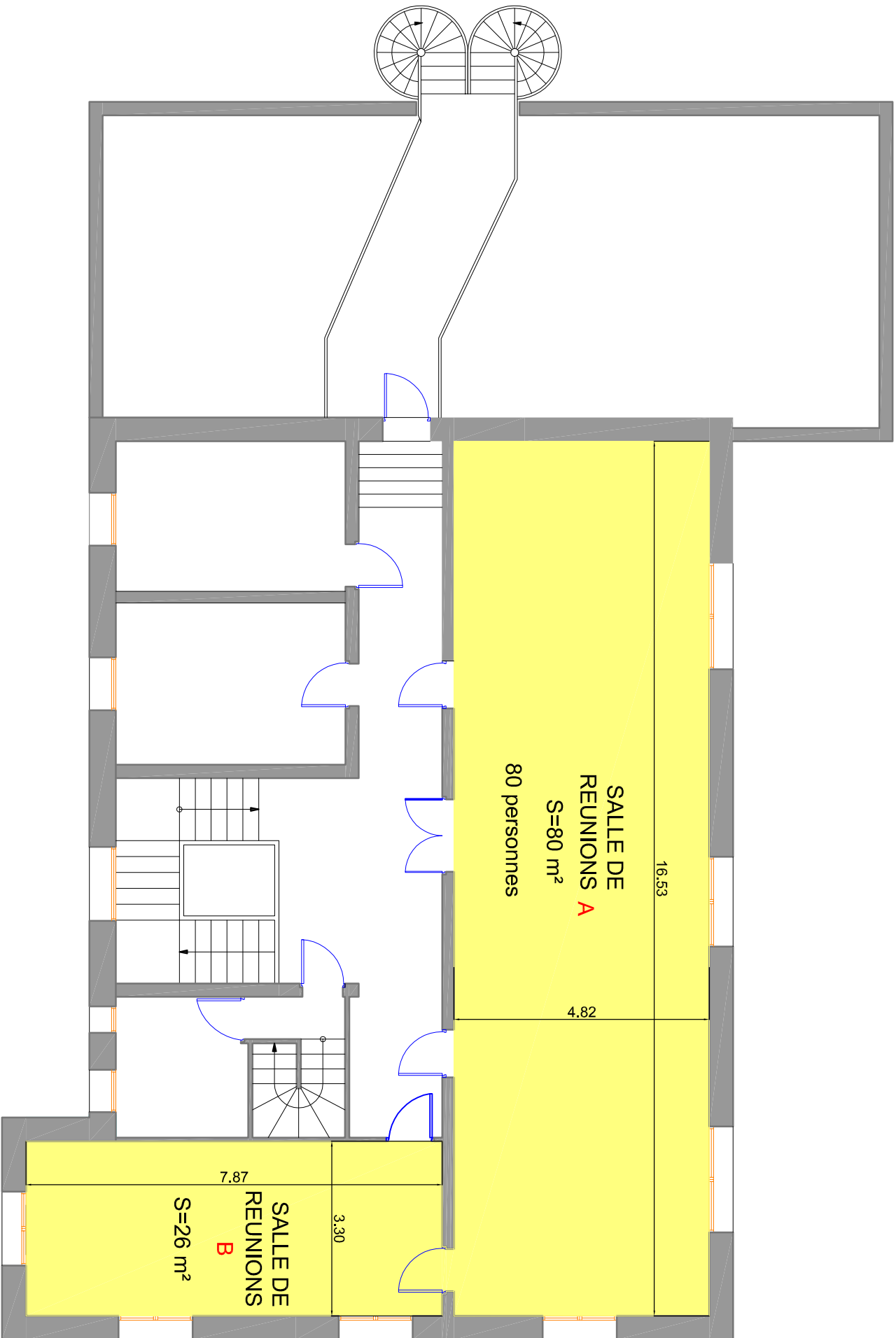
ETAGE 1
